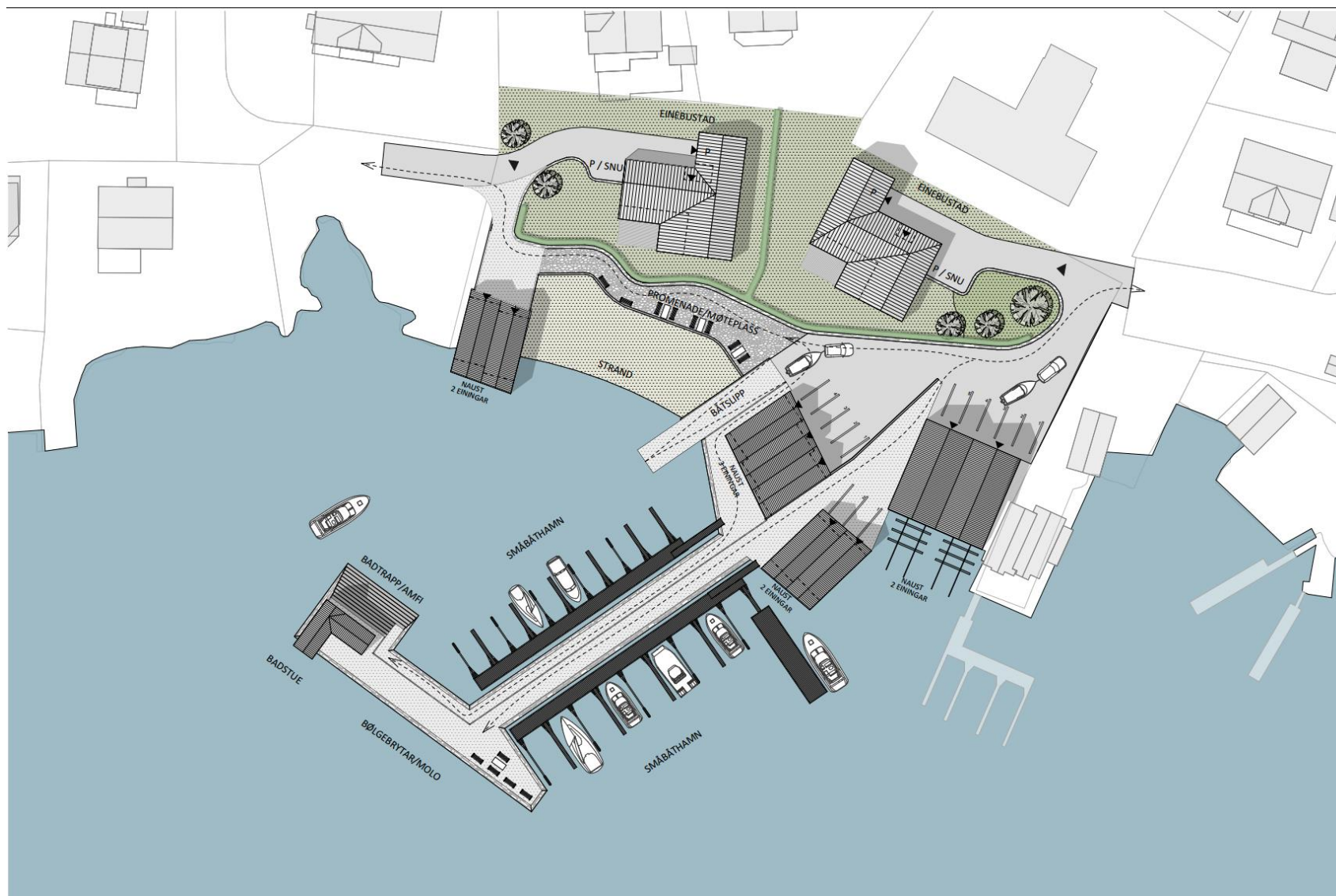
Figur 3: Illustrasjonsplan viser tenkt etablert situasjon. Utarbeida av Salt Arkitekter
